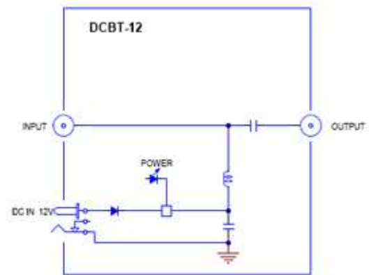
DCBT-12 ブロック図
